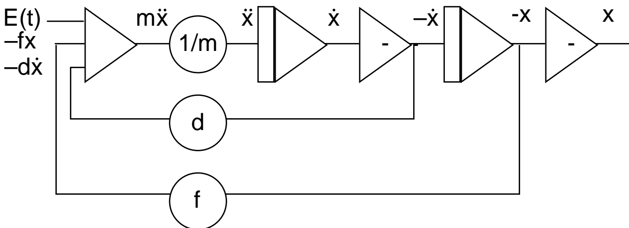
Bild 10.0.05: Schaltung DGI Radauslenkung
