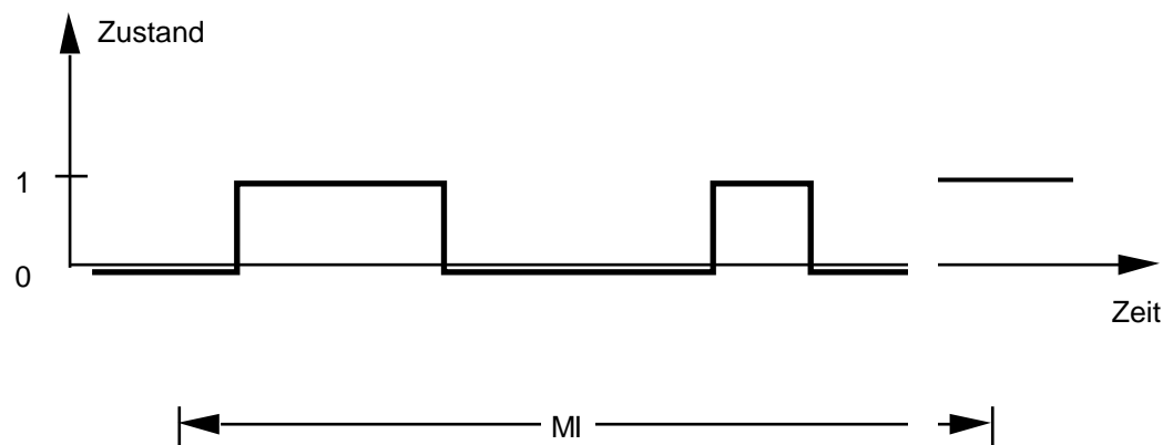
Abbildung 2.1.3: Sampling-Beobachtung CPU-busy-bit
