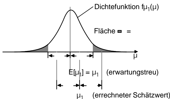
Abbildung 3.2.18: Dichtefunktion \tilde{\mu}_1 und Konfidenzintervall \mu^*_1 \pm
