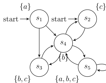
Abbildung 1: Transitionssystem TS
