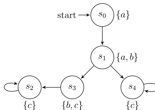
Abbildung 1: Transitionssystem TS_1
