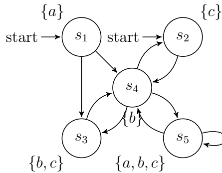
Abbildung 2: Transitionssystem TS_2
