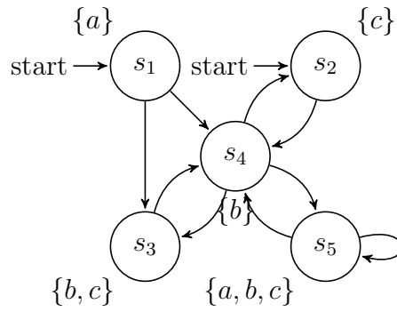
Abbildung 2: Transitionssystem TS
